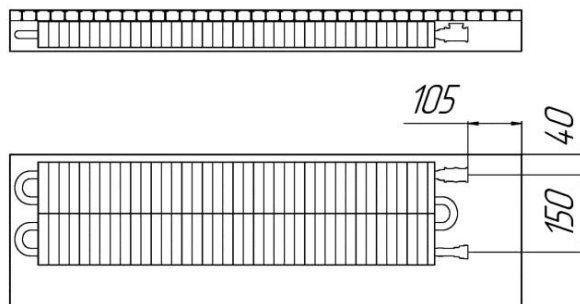
Расположение теплообменников в конвекторах Бриз шириной 300 (сечение)
