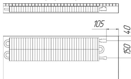
Расположение теплообменников в конвекторах Бриз шириной 380 (сечение)
